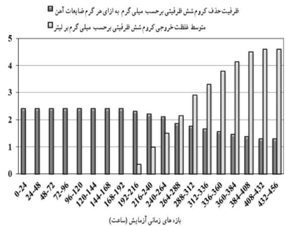
شکل ۸- ظرفیت حذف ضایعات آهن (RC SI ) و غلظت متوسط کروم (VI) خروجی در برابر زمان در pH=۲/۵
