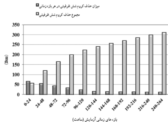
شکل ۵- میزان حذف کروم (VI) در برابر زمان در pH=۵/۱
