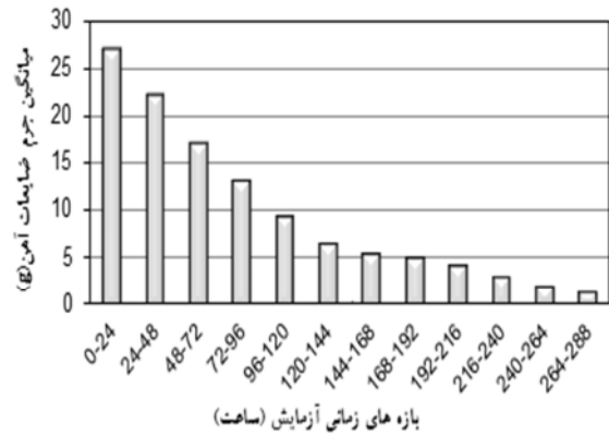
شکل ۱۲- میانگین جرم ضایعات آهن پر شده در pH=2
