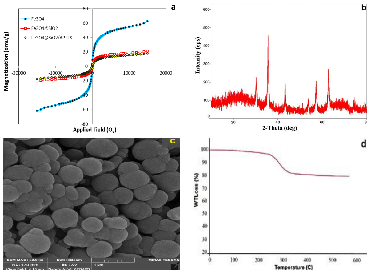
Fig. 3. a) VSM, b) XRD, c) SEM and d) TGA of \text{Fe}_3\text{O}_4@\text{SiO}_2/\text{APTES} nanoparticles شکل ۳- (a) VSM، (b) XRD، (c) SEM و (d) TGA نانوذرات \text{Fe}_3\text{O}_4@\text{SiO}_2/\text{APTES}
