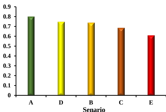
Fig. 4. Ranking of scenarios based on GFDM results شکل ۴- رتبه‌بندی سناریوها بر اساس نتایج GFDM
