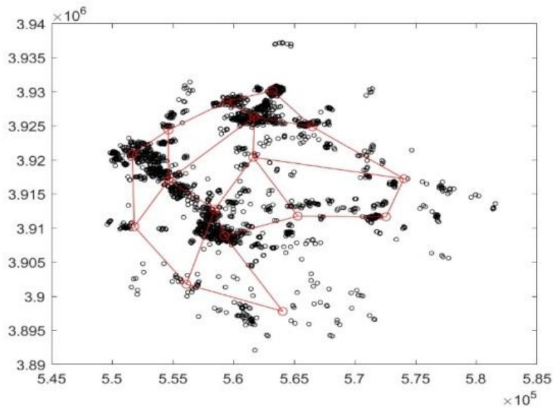
Fig. 3. SOM output in MATLAB environment
