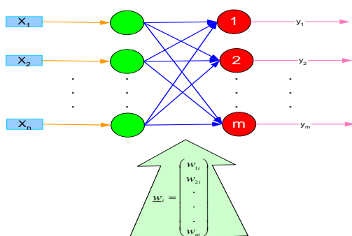
Fig. 3. Structural model of the two-dimensional Kohonen network شکل ۳- مدل ساختاری شبکه کوهون دوبعدی
