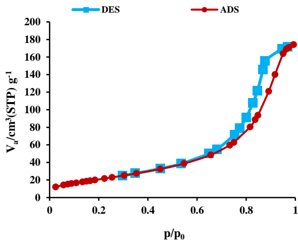
Fig. 6. N_2 absorption and desorption diagrams of photocatalyst شکل ۶- نمودارهای جذب و واجذب نیتروژن برای فوتوکاتالیست
