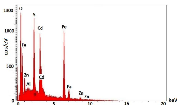
Fig. 4. EDX pattern of Fe_3O_4@BNPs@ZnS-CdS شکل ۴- الگوی EDX فوتوکاتالیست Fe_3O_4@BNPs@ZnS-CdS
