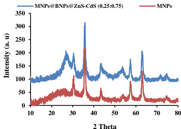
Fig. 1. XRD diagrams of Fe_3O_4@BNPs and Fe_3O_4@BNPs@ZnS-CdS شکل ۱- طیف فوتوکاتالیست Fe_3O_4@BNPs@ZnS-CdS
