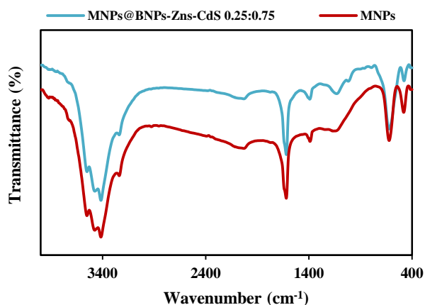
Fig. 2. FTIR spectra of MNPs and Fe_3O_4@BNPs@ZnS-CdS شکل ۲- طیف‌های مادون قرمز برای نانوذرات آهن و Fe_3O_4@BNPs@ZnS-CdS
