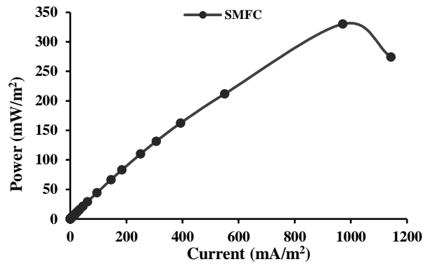
Fig. 6. Diagram of power density شکل ۶- نمودار چگالی توان راکتور
