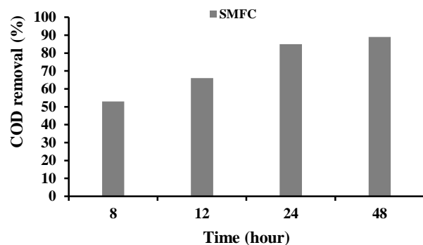
Fig. 11. COD removal efficiency at different times شکل ۱۱- کارایی حذف COD در زمان‌های مختلف
