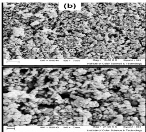
شکل ۱- تصویر SEM از نانوذرات دی‌اکسید منگنز
