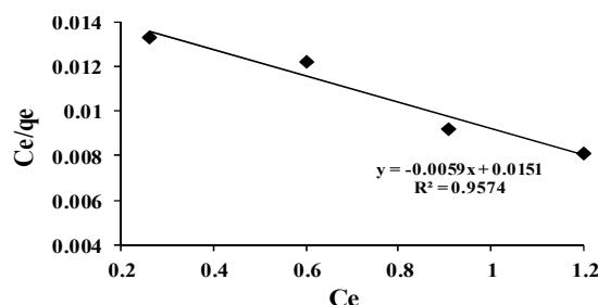
شکل ۱۰- نمودار ایزوترم لانگمیر جذب مس توسط نانوذرات دی‌اکسید منگنز
