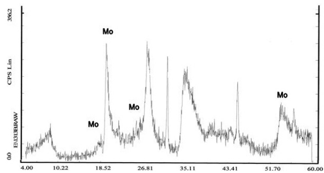
شکل ۲- الگوی XRD (pattern) از نمونه بنتونیت سدیم دار
