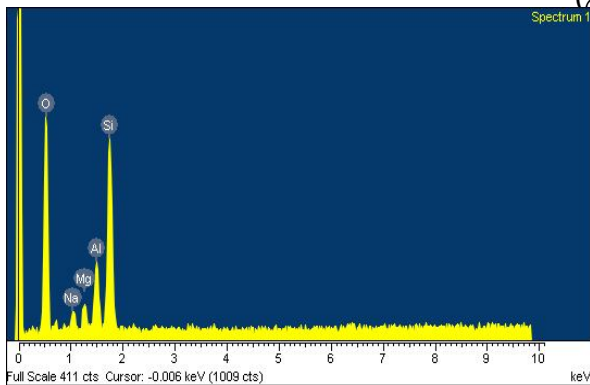
شکل ۵- تصاویر و آنالیزهای حاصل از SEM با سیستم EDS الف- گل قرمز خام، ب- گل قرمز تعدیل شده، ج- بنتونیت خام، د- بنتونیت سدیم دار شده
