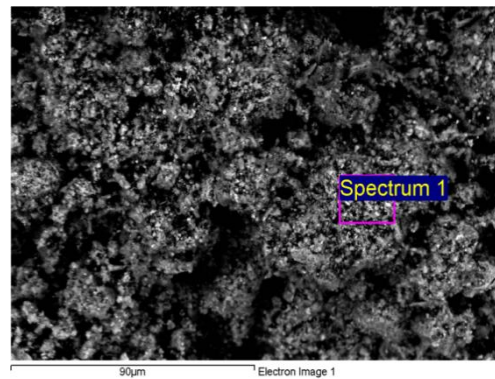
شکل ۶- تصاویر و آنالیزهای حاصل از SEM با سیستم EDS الف- رس پیلارد ، ب- رس پیلارد جذب کننده کادمیم
