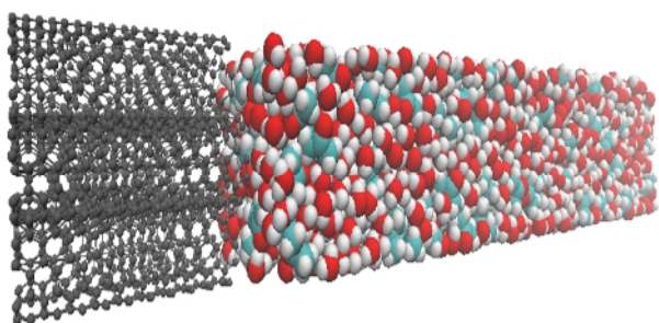
Fig. 3. A snapshot of the simulation box with the size of 18 \times 18 \times 230 \text{ \AA}^3 شکل ۳- نمای از جعبه شبیه‌سازی به ابعاد 18 \times 18 \times 230 آنگستروم مکعب
