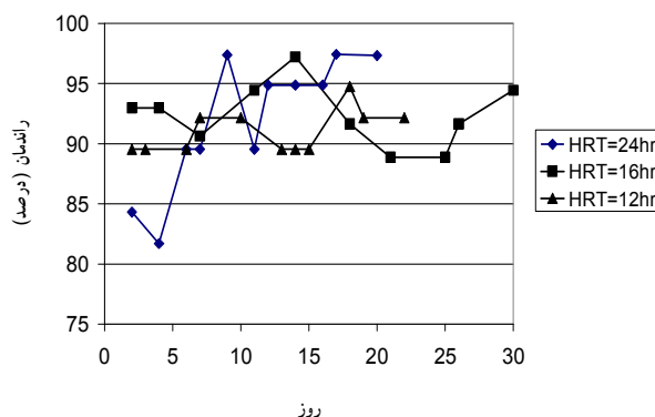
شکل ۵- تغییرات کارایی حذف آلاینده در طول روزهای آزمایش (COD in = ۱۵۰۰ میلی گرم بر لیتر)
