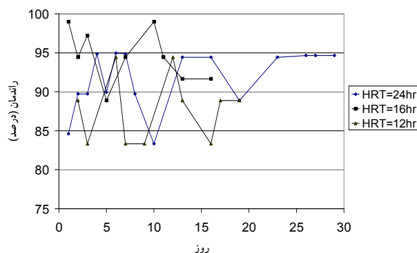
شکل ۴- تغییرات کارایی حذف آلاینده در طول روزهای آزمایش (COD in = ۷۵۰ میلی گرم بر لیتر)
