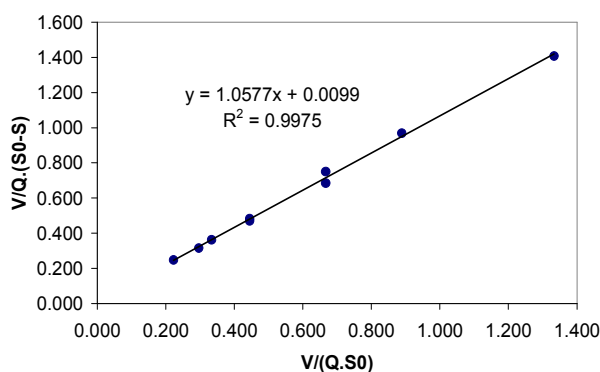
شکل ۱۰- نمودار رسم شده جهت بررسی مدل استوور-کن کانن
