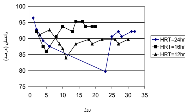
شکل ۶- تغییرات کارآیی حذف آلاینده در طول روزهای آزمایش (۲۲۵۰ میلی‌گرم بر لیتر = COD_{in} )
