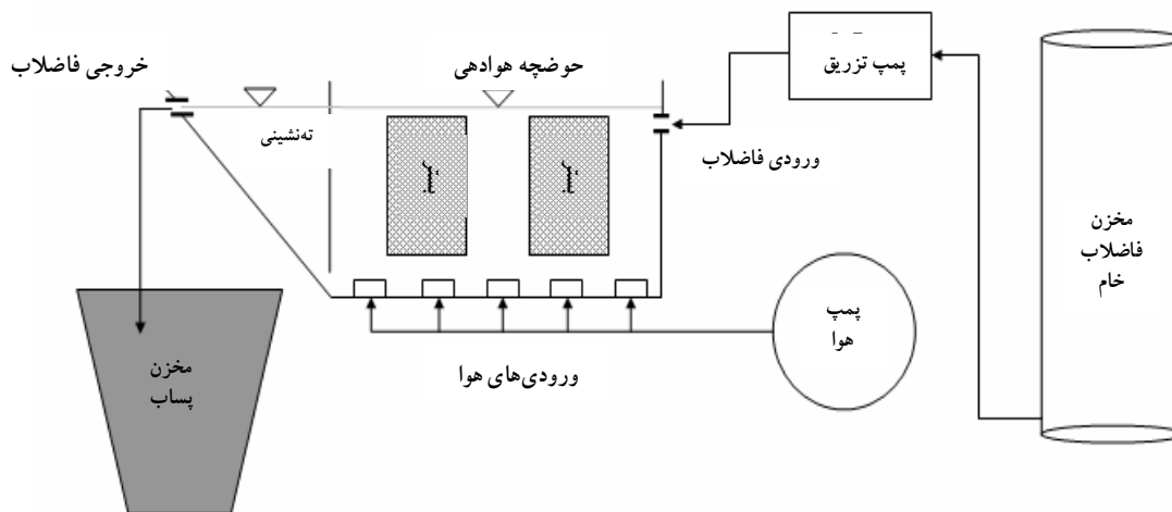
شکل ۱- نمای شماتیک راکتور لجن فعال دارای بستر ثابت رشد میکروبی
