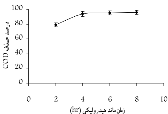
شکل ۲- میانگین بازده حذف COD در زمان‌های ماند ۲، ۴، ۶، ۸ ساعت و غلظت ورودی ۵۰۰ میلی‌گرم در لیتر در شرایط پایدار
