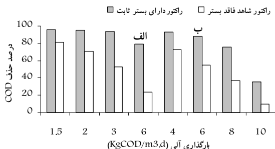
شکل ۴- مقایسه بازده حذف COD در راکتورهای لجن فعال دارای
