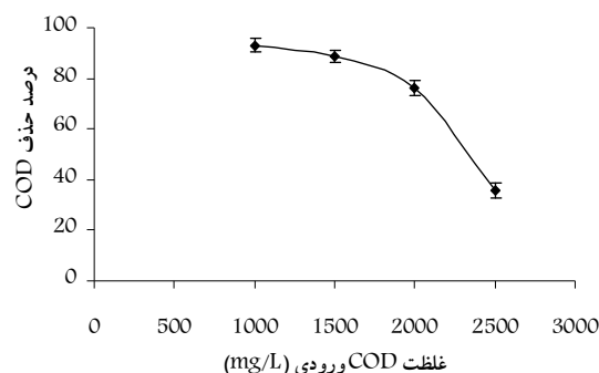
شکل ۳- میانگین بازده حذف COD در غلظتهای ورودی ۱۰۰۰ تا ۲۵۰۰ میلی‌گرم در لیتر و زمان ماند هیدرولیکی ثابت ۶ ساعت در شرایط پایدار
