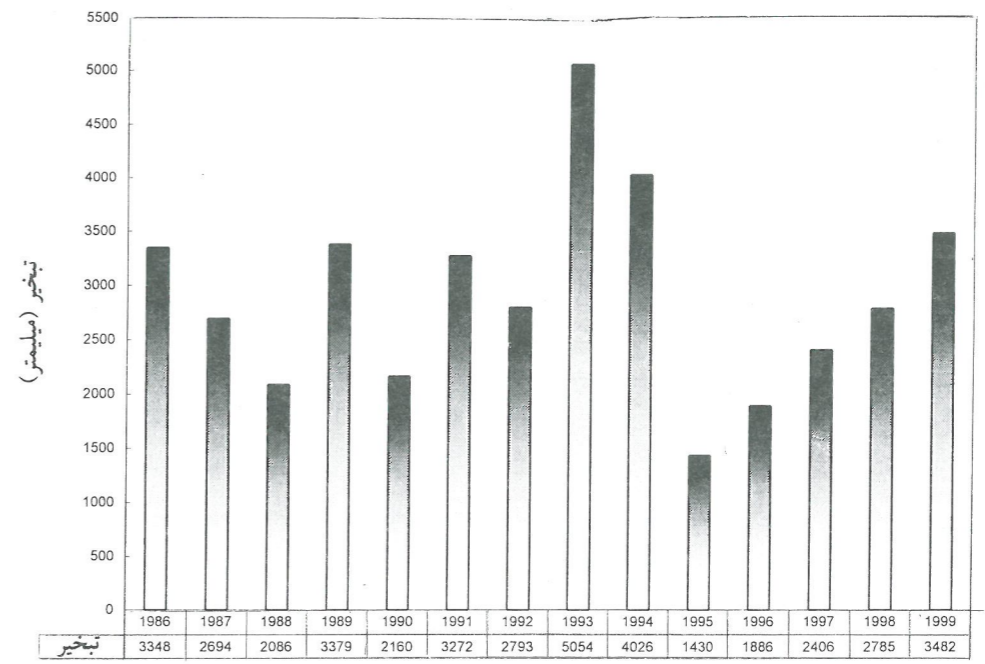
شکل ۳- میزان تبخیر سالانه با استفاده از بیلان آبی.
