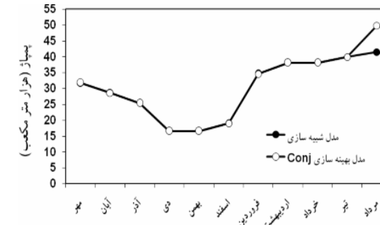
شکل ۱۲- تغییرات میزان پمپاژ از سه سلول نمونه در مدل‌های شبیه‌سازی و بهینه‌سازی
