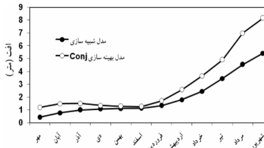
شکل ۱۳- تغییرات میزان افت تراز در سه سلول نمونه در مدل‌های شبیه‌سازی و بهینه‌سازی
