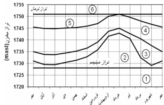
شکل ۶- منحنی فرمان بهره‌برداری از مخزن سد کینه ورس
