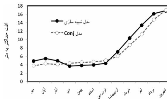
شکل ۱۱- تغییرات افت ماکزیم ماهانه در سلولهای شبکه در مدل های شبیه سازی و بهینه سازی
