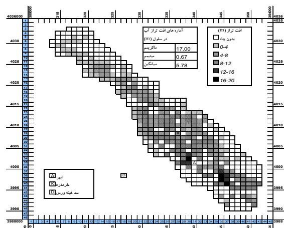
شکل ۹- پراکنده مکانی افت تراز سلولهای شبکه براساس نتایج مدل بهینه سازی تلفیقی در انتهای شهریورماه
