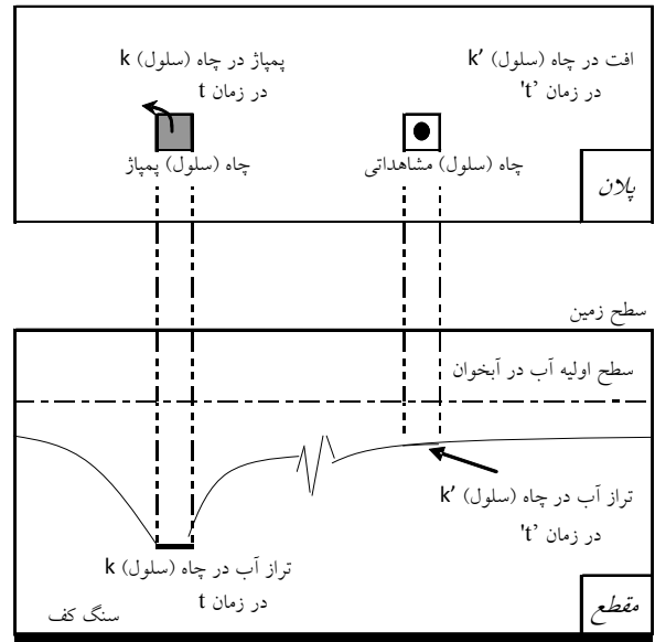
شکل ۱- مفهوم ضریب پاسخ واحد
