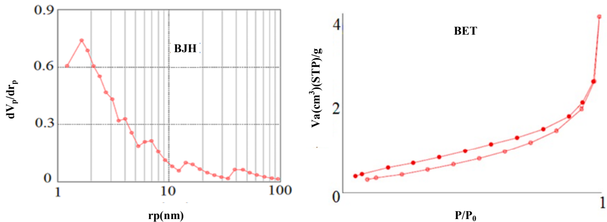
Fig. 3. The N_2 adsorption-desorption isotherm and the BJH curve شکل ۳- منحنی جذب-واحد نیتروژن و منحنی بدست آمده از آنالیز BJH
