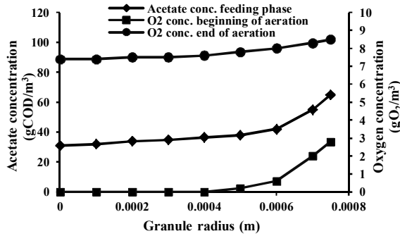
Fig. 2. The simulated results of the profile of acetate and dissolved oxygen concentrations inside the granules شکل ۲- عمق نفوذ اکسیژن و استات در داخل گرانول با مدل
