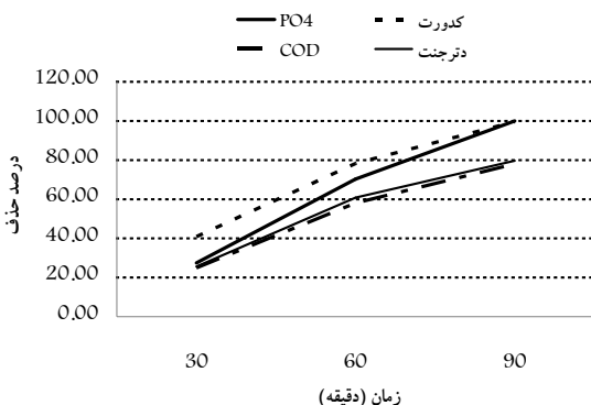
شکل ۳- درصد حذف آلاینده‌ها در طی فرایند EC در شرایط بهینه ولتاژ و pH با الکتروود آلومینیوم
