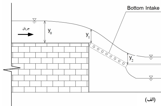
شکل ۴- الف- مقطع طولی و ب- پلان کف مشبک نصب شده داخل کانال و پارامترهای هندسی مدل
