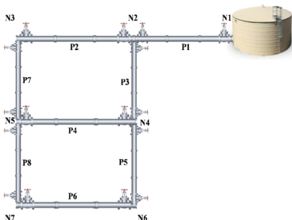
Fig. 4. The two-loop water distribution system assessed in WDSR-Min model شکل ۴- شبکه دو حلقه‌ای مورد بررسی در مدل WDSR-Min
