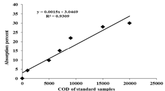
Fig. 1. COD standard curve شکل ۱- منحنی استاندارد COD
