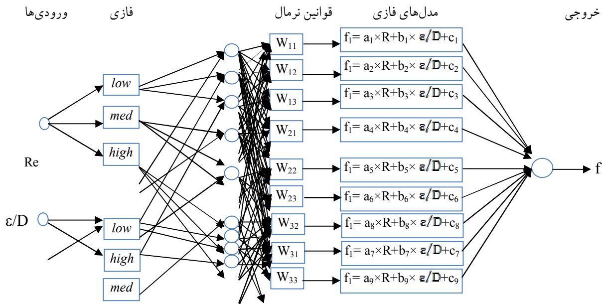
شکل ۱- سیستم استنتاجی فازی تاکاگی - سوگنو شامل دو متغیر ورودی R و D/\varepsilon و یک خروجی f
