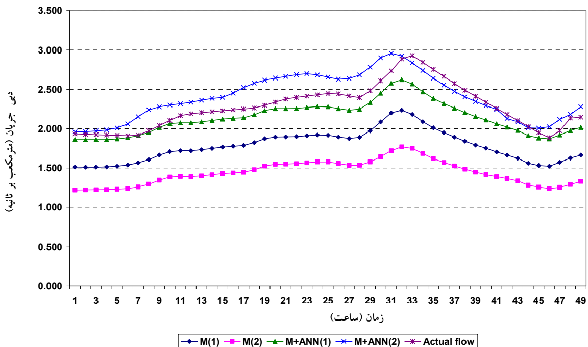
شکل ۶- نتایج مدل‌های هیدرودینامیکی و شبکه عصبی مصنوعی در مراحل اول و دوم برای یک محدوده زمانی دبی کم جریان
