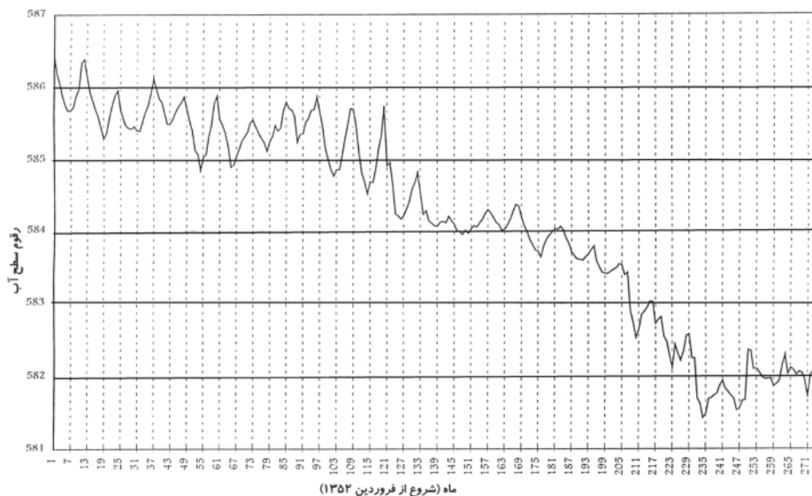
شکل ۴- هیدروگراف واحد آبخوان
