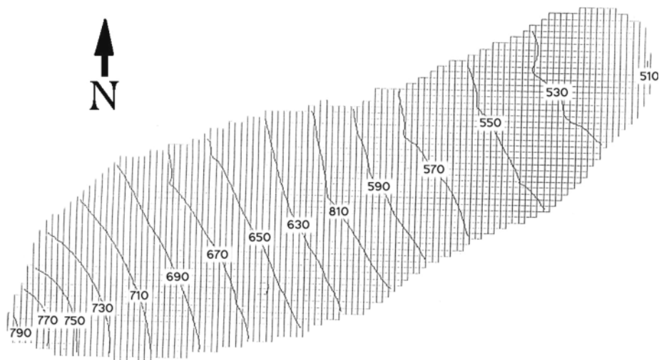
شکل ۵- نقشه تراز سطح آب زیرزمینی پس از واسنجی مدل در حالت ماندگار
