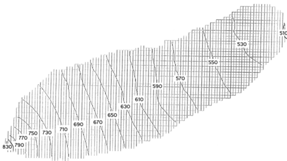
شکل ۸- نقشه خطوط تراز سطح ایستابی برای دوره زمانی ۵۰
