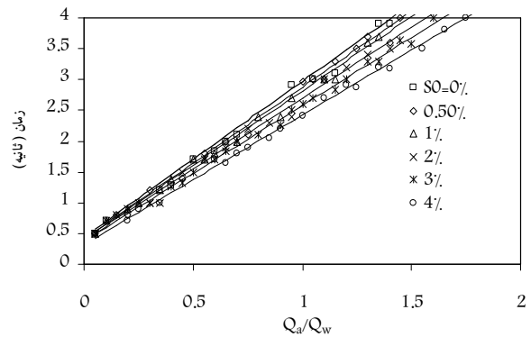
شکل ۷- منحنی تغییرات متوسط پیروید موج در شیب های مختلف بر حسب نسبت دبی هوا و آب
