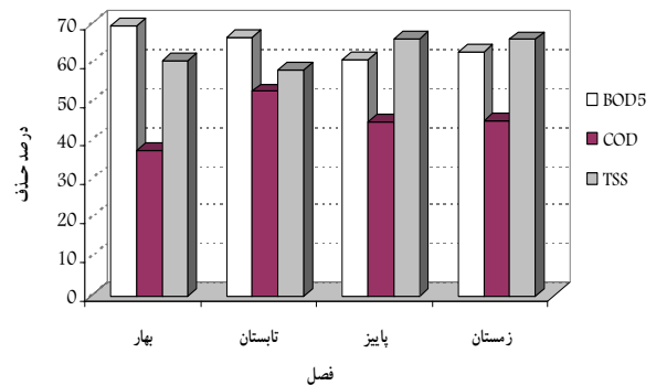
شکل ۴- درصد حذف BOD_5 ، COD و TSS در فصل‌های مختلف
