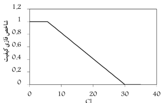
شکل ۳- پخش فازی غلظت پارامتر شیمیایی Cl و تغییرات شاخص آن به منظور آب آشامیدنی (دوزنقه ناقص)
