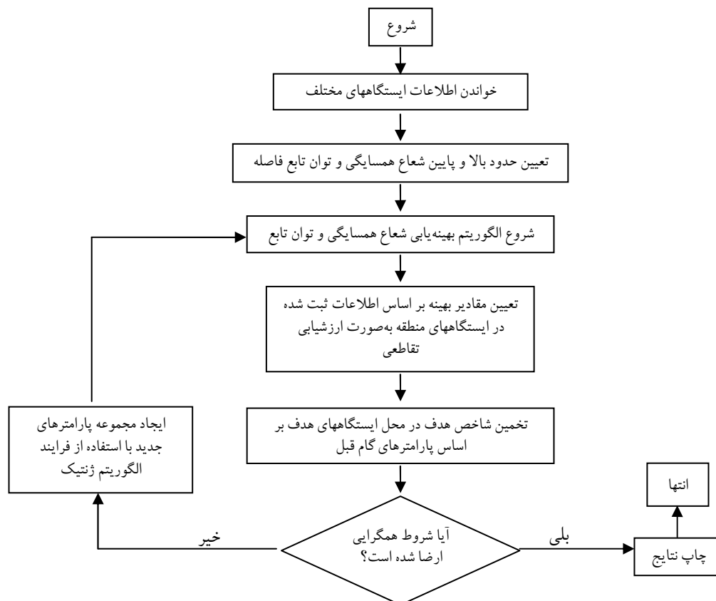
شکل ۵- نمودار گردش بهینه‌سازی معکوس وزن دار فاصله توسط الگوریتم ژنتیک در منطقه
