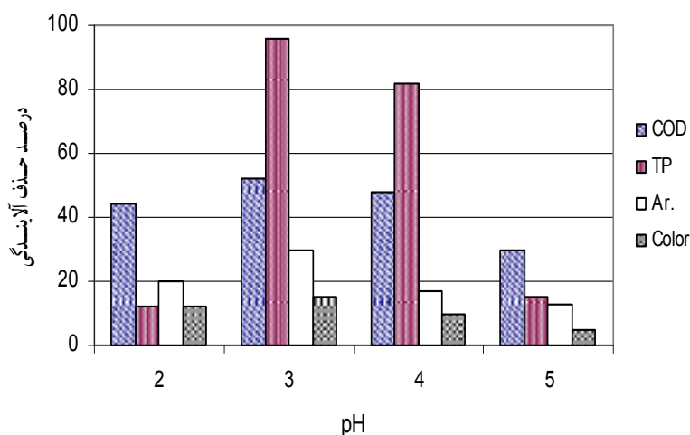
شکل ۳- تأثیر pH بر راندمان حذف شاخصهای آلاینده‌گی
