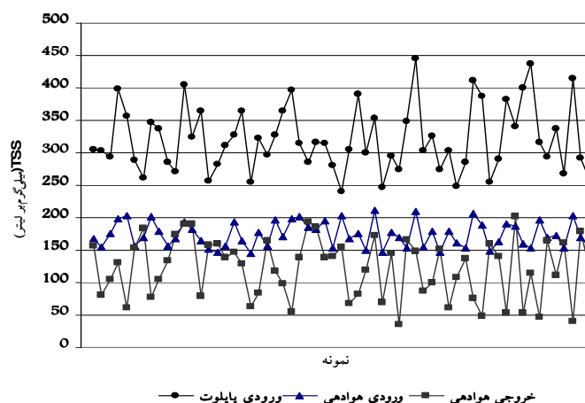
شکل ۴ - تغییرات TSS فاضلاب در بخشهای مختلف پایلوت
