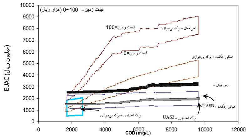
شکل ۳- تحلیل حساسیت EUAC نسبت به ورودی و قیمت زمین
