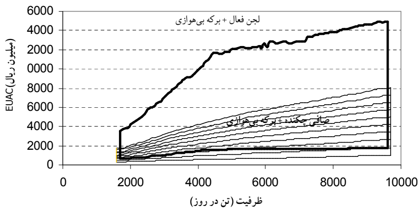
شکل ۴- تحلیل حساسیت EUAC نسبت به ورودی و ضریب تولید پساب
