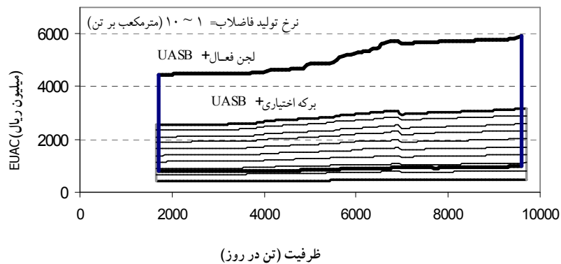
شکل ۳- تحلیل حساسیت EUAC نسبت به ورودی و قیمت زمین
