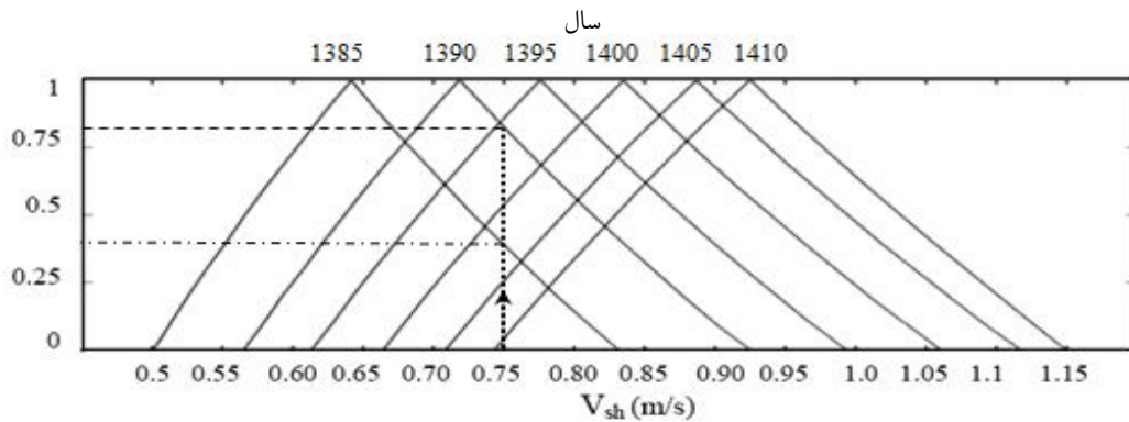
شکل ۹- سرعت شستشو در مجرای شماره دو برای سالهای مختلف بهره‌برداری
