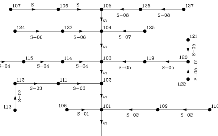
شکل ۳- پلان شبکه جمع‌آوری فاضلاب مورد مطالعه
