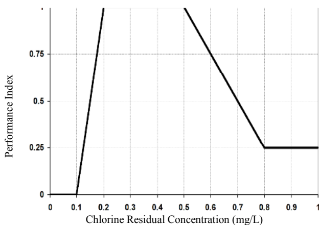
Fig. 1. Penalty curve of the residual free Chlorine (Coelho 1996) - منحنی جریمه برای کلر آزاد باقیمانده (Coelho 1996)
