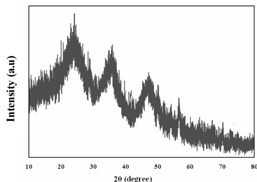
Fig. 3. XRD pattern of TiO 2 -PAA-Ch شکل ۳- الگوی XRD مربوط به نمونه TiO 2 - Polyacrylamide/Chitosan
