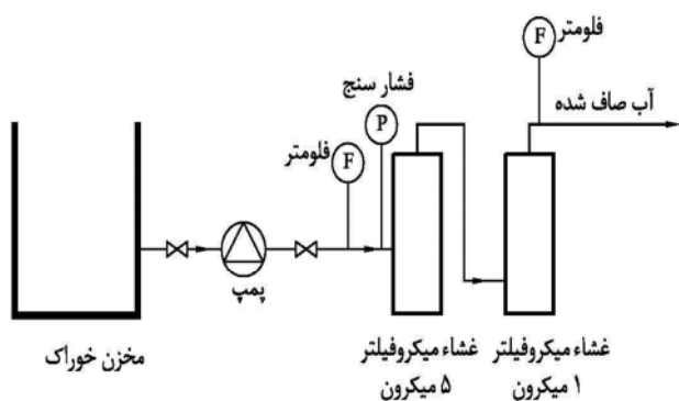
شکل ۱- فلودیگرام پایلوت میکروفیلتراسیون
