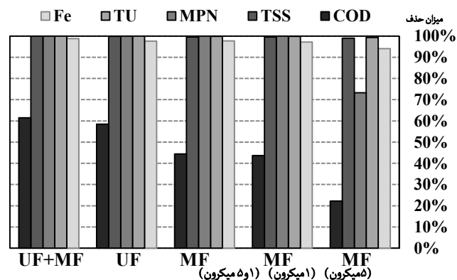
فرایند تصفیه
