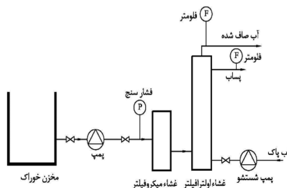
شکل ۲- فلودیگرام پایلوت اولترافیلتراسیون
