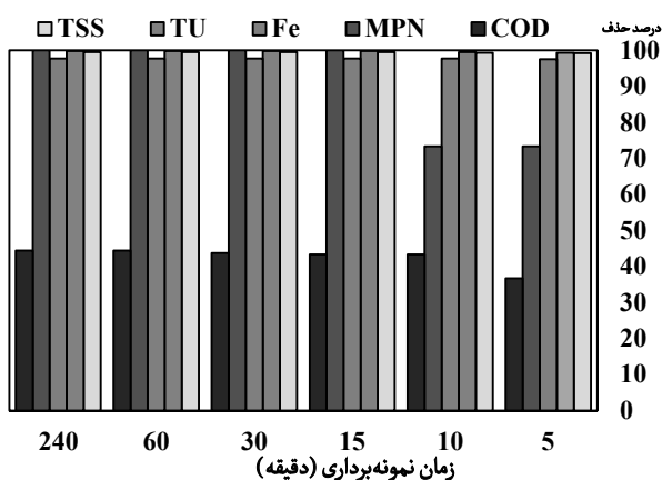
شکل ۵- نتایج حاصل از عملکرد غشای میکروفیلتر ترکیبی ۱ و ۵ میکرون، در کاهش پارامترهای مورد اندازه‌گیری آب حاصل از شستشوی معکوس فیلترهای شنی
