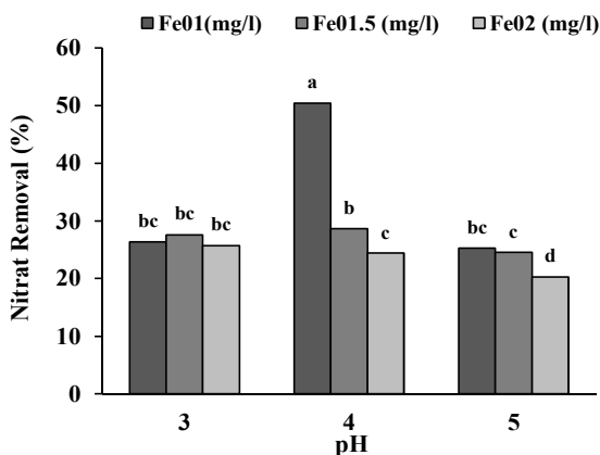
Fig. 7. Fe 0 nano-particles × pH interaction effect on nitrate removal form water containing 30 mg/L nitrate شکل ۷- اثر متقابل نانوذرات آهن صفر و pH بر راندمان حذف نیترات از آب حاوی ۳۰ میلی‌گرم در لیتر نیترات
