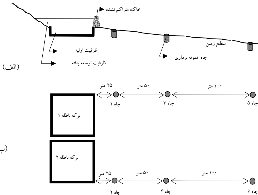
شکل ۱- نمای منطقه مورد مطالعه الف- مقطع عرضی ب- پلان
