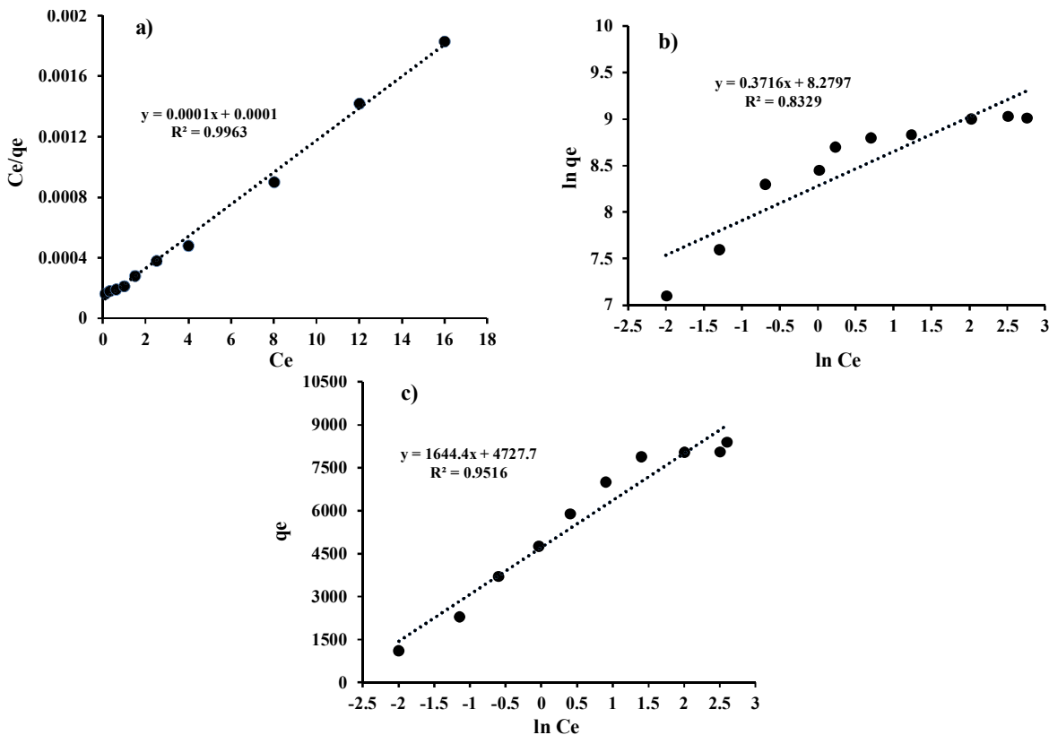
Fig. 8. Fit of a) Langmuir, b) Freundlich and c) Temkin isotherms data for the adsorption of Cr^{3+} onto the MGO-IDA شکل ۸- نمودارهای مدل ایزوترمی (a) لانگمیر، (b) فروندلیچ و (c) تمکین در فرایند جذب کروم بر روی جاذب اکسید گرافن مغناطیسی عامل دار شده با ایمینو دی استیک اسید
