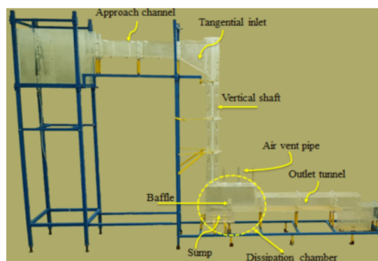
Fig. 2. Experimental model of vortex drop structure شکل ۲- مدل آزمایشگاهی سازه ریزشی گردابی
