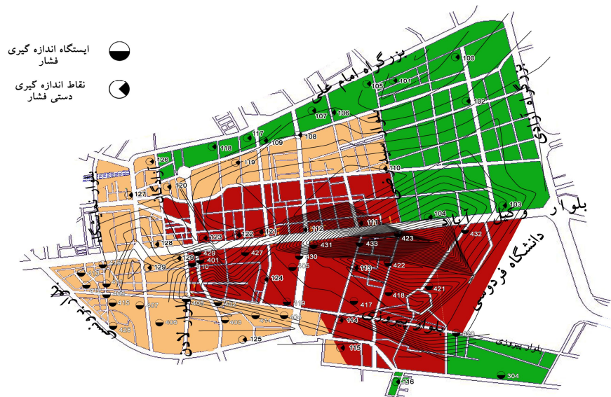
شکل ۲- کروکی محدوده‌ها و خطوط هم فشار در منطقه مطالعاتی [۱۶]
